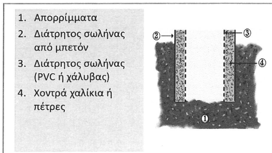
Εικόνα 5,6: Τυπική Διατομή κατακόρυφου φρέατος απαγωγής βιοαερίου
